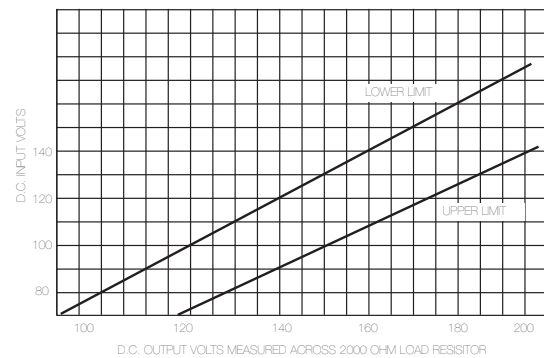
Fig. 11 D.C./A.C. Inverter (Art No. 410A21535).
